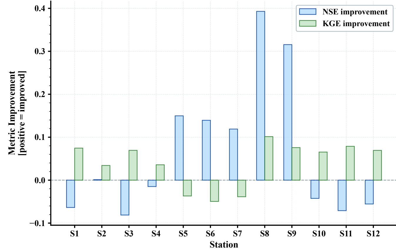
(d) NSE & KGE Improvement
